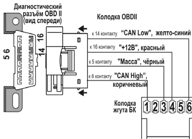
Рис.2 Схема подключения БК «ШТАТ Х1-Г»
